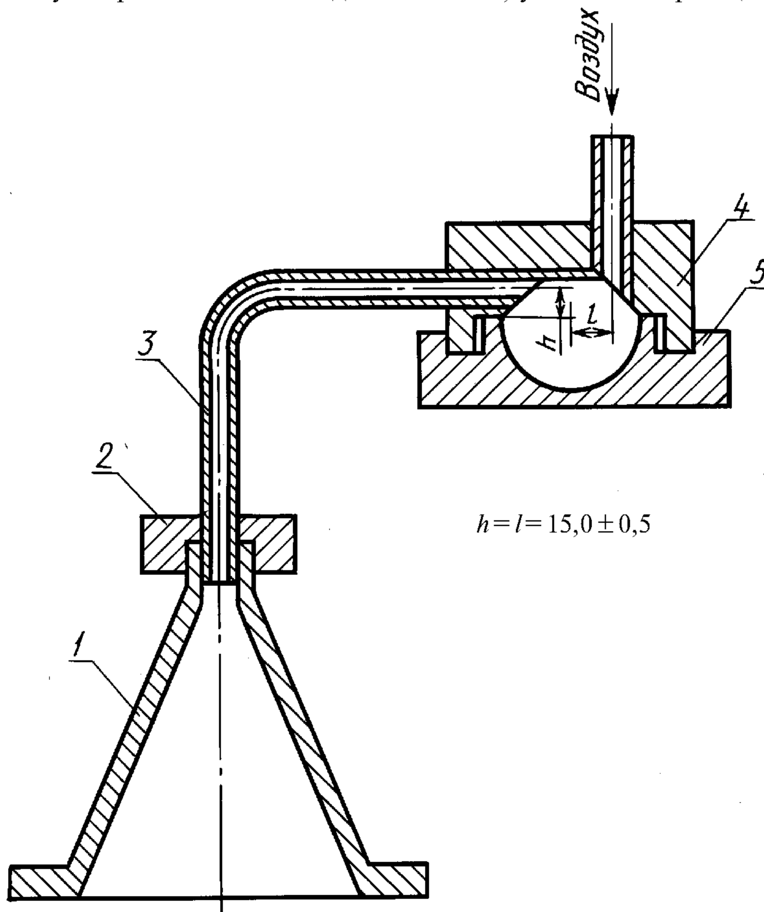
1 — конус; 2 — гайка накидная; 3 — патрубок; 4 — корпус форкамеры; 5 — доньшко
